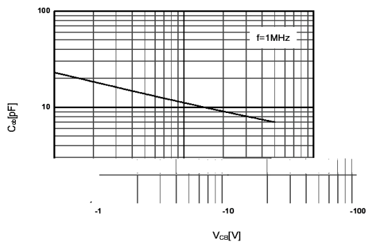
C_{ob} - V_{CB}
